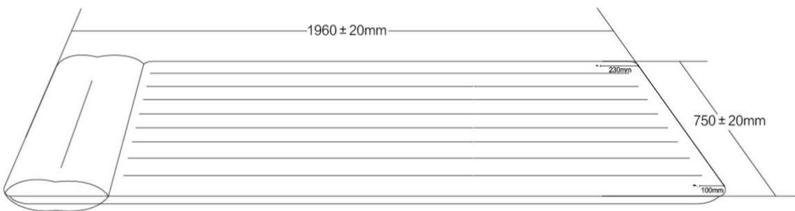
图2 充气状态
