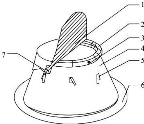
软体贮水罐收拢状态
